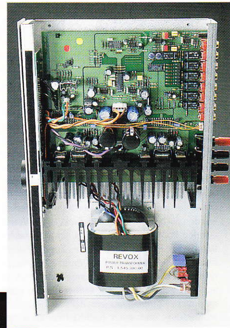
Bild 3 Sauberes Innenleben: Exemplarisch beweist der Verstärker S25 die sehr gute Verarbeitungsqualität der Elegance-Linie. Uppig dimensionierter Kühlkörper und streuarmer Hochleistungstransformator.
